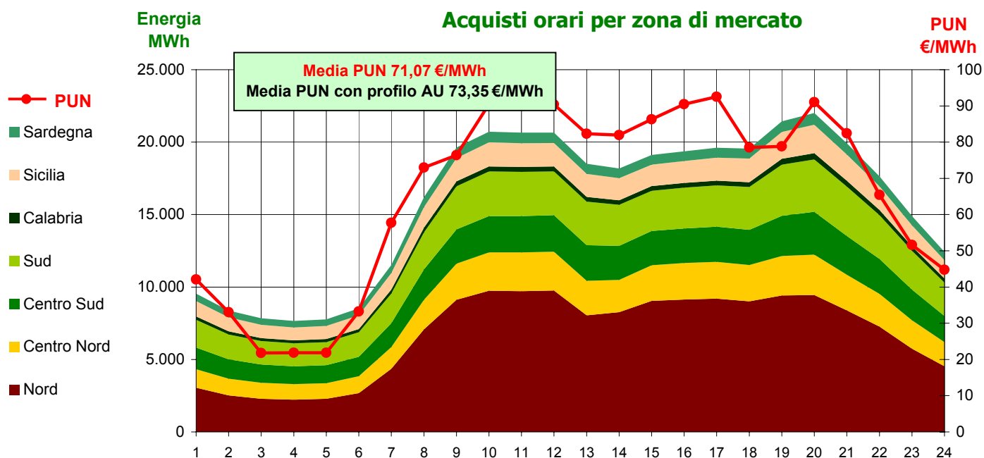
PUN vs PGn (€/MWh)
